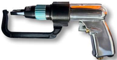
Perslucht puntlasfreemachine PS 25
