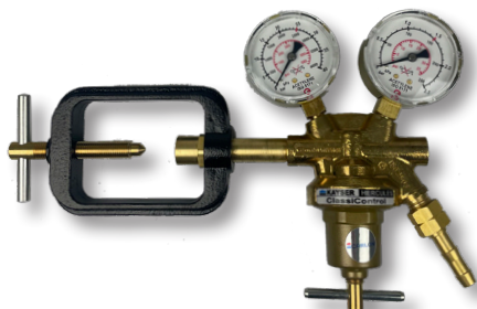
Reduceerventiel Acetyleen
